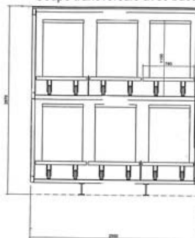
Coupe transversale avec bacs
